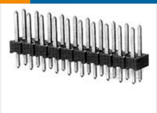
TE 产品编号826942-5 5P MOD2 STIFT LEI
