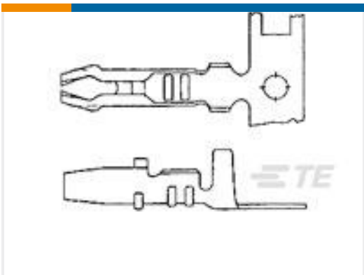
TE 产品编号172769-1 AMP-IN 24-20 AWG LP
