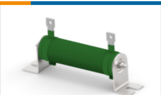
TE 产品编号1879456-1 线绕电阻器：矿物，2.5 Kw
