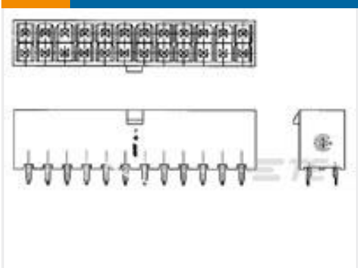
TE 产品编号1586038-8 8P VRT HDR VAL-U-LOK V0
