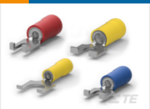
TE 产品编号2-320861-1 PIDG 带凸缘叉形舌片端子
