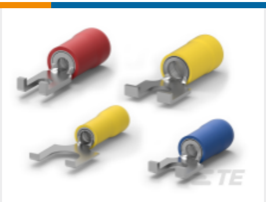
TE 产品编号1-325150-0 PIDG 带凸缘叉形舌片端子
