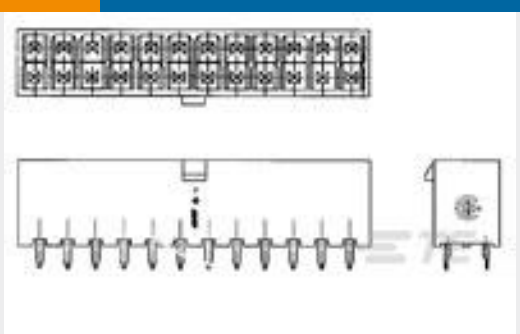
TE 产品编号1586038-8 8P VRT HDR VAL-U-LOK V0
