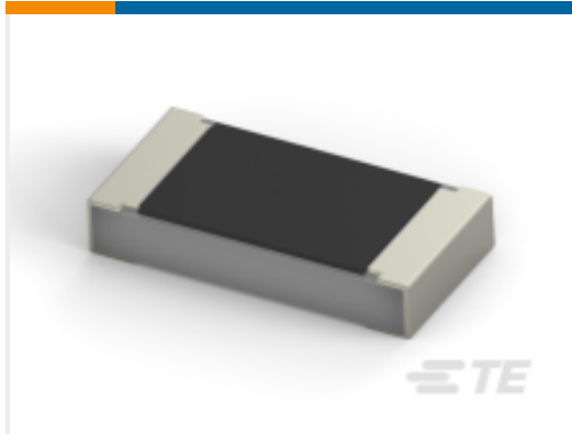
TE 产品编号1-2176230-5 SMD 功率电阻器：3 瓦特，5% Tol
