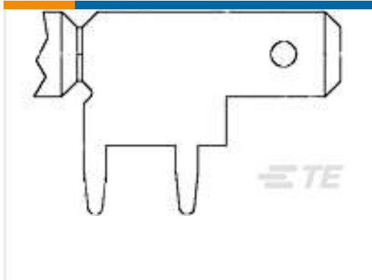
TE 产品编号1217156-1 187 FASTON,PCB TAB,TNBR
