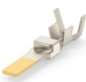
TE 产品编号 CAT-D9934-A83 Dynamic 5000 矩形公端子
