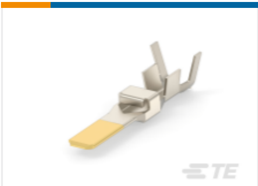
TE 产品编号84695-1 Dynamic 5000 矩形公端子
