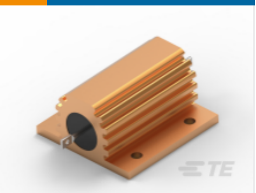
TE 产品编号1-1625995-7 功率电阻器：铝壳体，HSA
