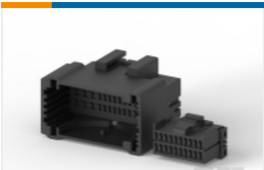
TE 产品编号176119-6 MULTILOCK™, 连接器壳体
