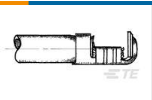
TE 产品编号170023-1 BUTTON CONTACT
