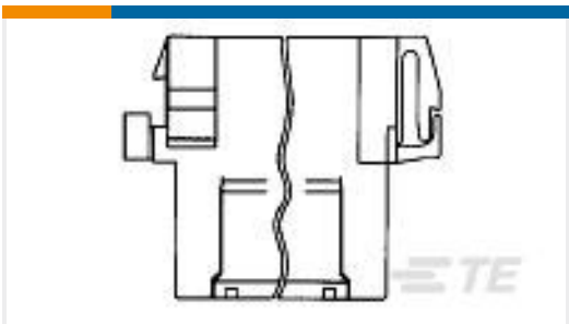
TE 产品编号1-929505-7 TAB HSG .110 (2.8 MM) HSG TAB
