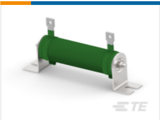
TE 产品编号1879446-1 线绕电阻器：矿物，2.5 Kw
