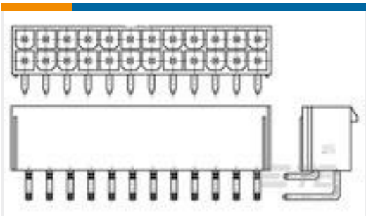
TE 产品编号1-1586041-0 10P VAL-U-LOK R/A HDR V2
