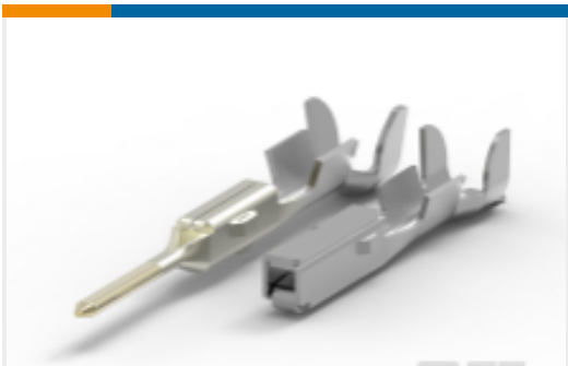
TE 产品编号179417-1 MULTILOCK，母端和公端
