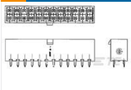
TE 产品编号1586038-8 8P VRT HDR VAL-U-LOK V0
