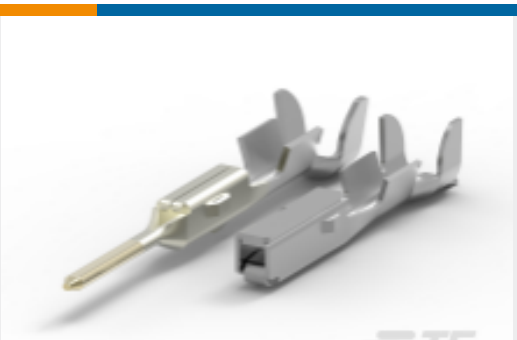
TE 产品编号917067-6 MULTILOCK，母端和公端
