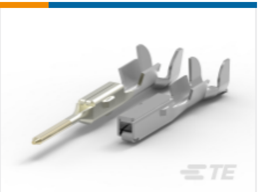
TE 产品编号1-368088-1 MULTILOCK，母端和公端
