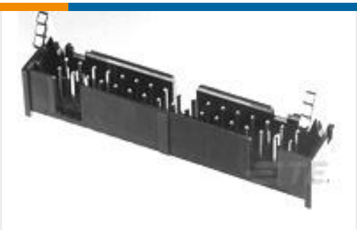
TE 产品编号1-1761608-1 IDC LOW PRO HDR 34P VERT SHT L
