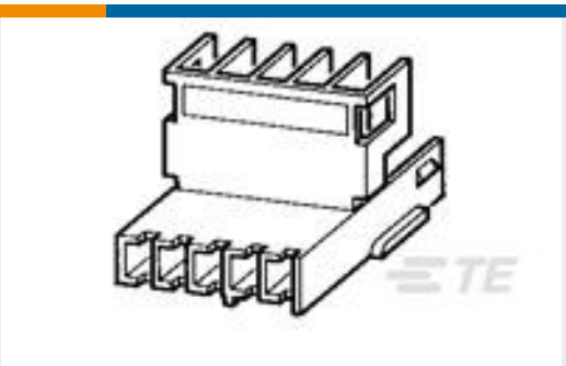
TE 产品编号1394005-1 MQS，连接器壳体
