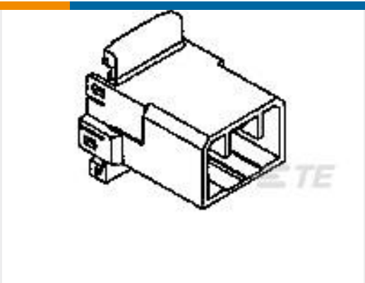
TE 产品编号1-174936-1 070 MLC W-W CAP HSG 20P F/A
