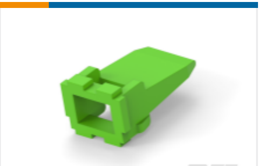
TE 产品编号2600032-1 4CCT ML-XT RECEPT WEDGELOCK GREEN
