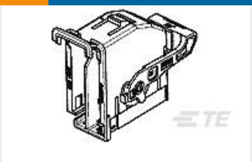
TE 产品编号284138-1 18 POS. FRAME ASS'Y 3,5 MM PIT
