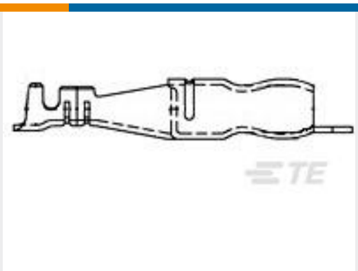
TE 产品编号444154-2 SHUR PLUG 180 0.5-1.0MM2 0.45X27.6 PTPBR
