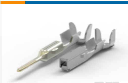
TE 产品编号175275-2 MULTILOCK，母端和公端
