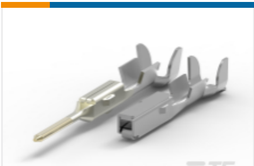
TE 产品编号284087-2 MULTILOCK，母端和公端
