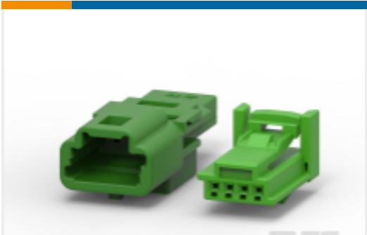
TE 产品编号1612802-1 TH/.025 连接器系统，壳体
