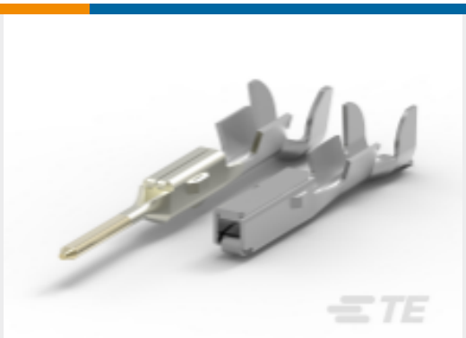
TE 产品编号2109005-1 MULTILOCK，母端和公端
