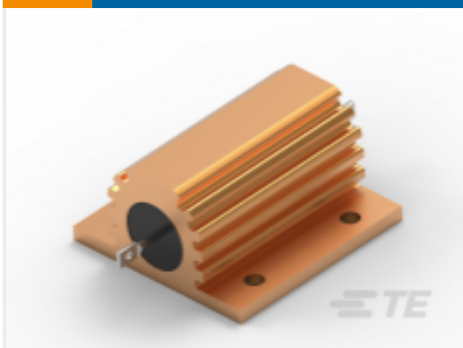
TE 产品编号2-1625963-4 功率电阻器：铝壳体，HSA
