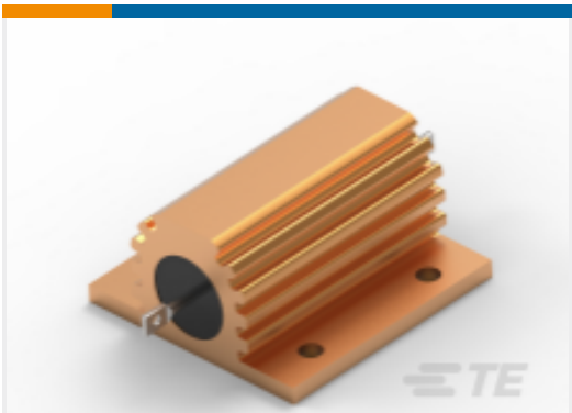
TE 产品编号1625984-1 功率电阻器：铝壳体，HSA
