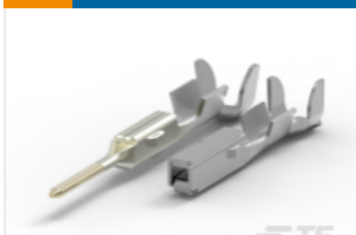
TE 产品编号173631-7 MULTILOCK , 母端和公端
