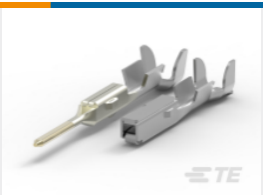
TE 产品编号173681-1 MULTILOCK，母端和公端
