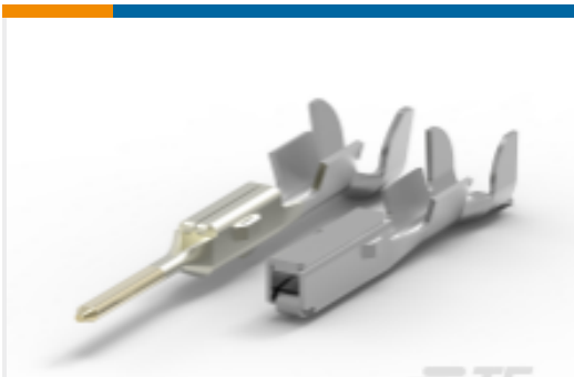
TE 产品编号173645-1 MULTILOCK，母端和公端
