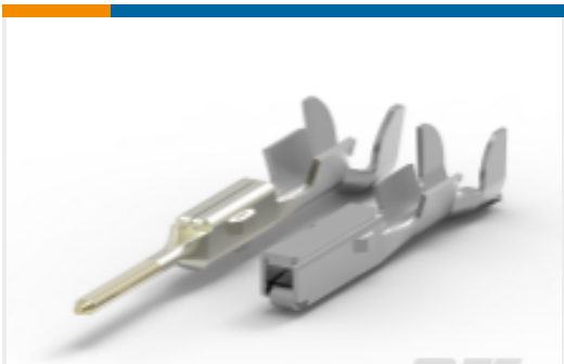
TE 产品编号173631-1 MULTILOCK · 母端和公端
