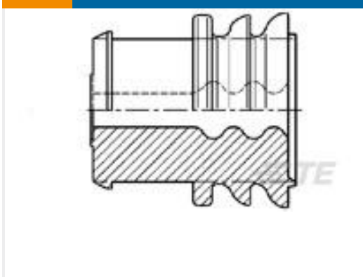
TE 产品编号963244-1 EINZELDRAHTDICHTUNG
