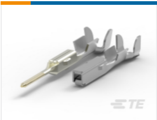
TE 产品编号1743654-1 MULTILOCK，母端和公端
