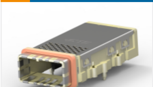
TE 产品编号2149733-1 CXP 母端套件
