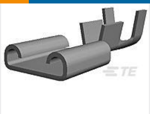
TE 产品编号1-280001-1 250 FASTON,REC.,14-17 AWG,BR
