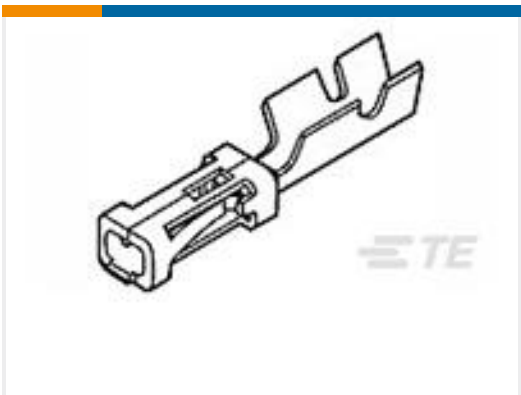
TE 产品编号102918-1 MOD IV RECP PLTD 30 SEL
