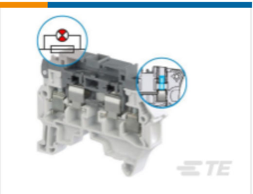
TE 产品编号1SNK508413R0000 ZS4-SF1-R2
