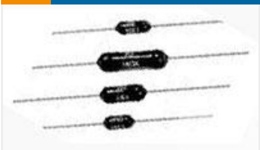
TE 产品编号1879664-6 H8 1K3 0.1% 15PPM
