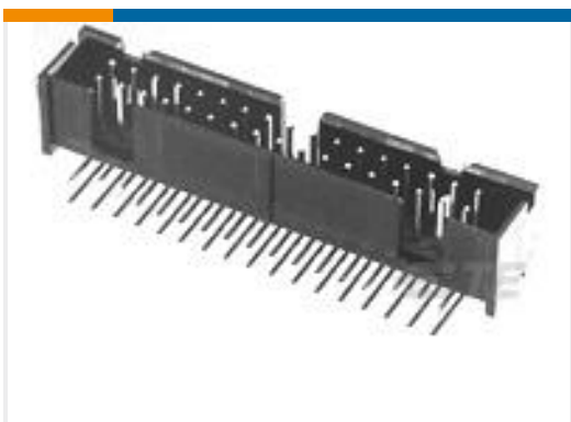
TE 产品编号103310-1 010 LOPRO HDR RA 15DP
