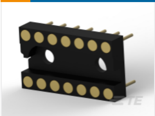
TE 产品编号3-1571550-2 DIP 插座：标准，自动车床，封闭式，镀金
