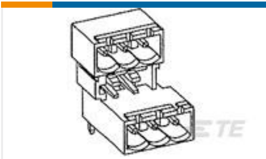
TE 产品编号1776166-6 6P TERMI-BLOK HDR, HIGH TEMP
