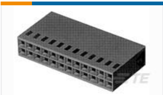
TE 产品编号86264-4 52 MODIV HSG COMP DR .100 EARS
