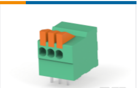
TE 产品编号1-2834016-3 3POS 2.54MM SES CONN.
