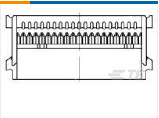
TE 产品编号3-1437021-4 609-3441=FSKT IDC S 34 30AU PL
