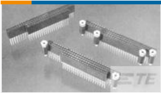
TE 产品编号1375796-3 ASSY, 64/40 POS PC104 LF
